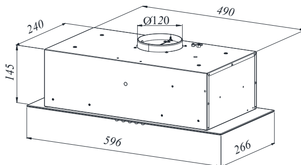
Рис. 2. Схема з розмірами моделі
