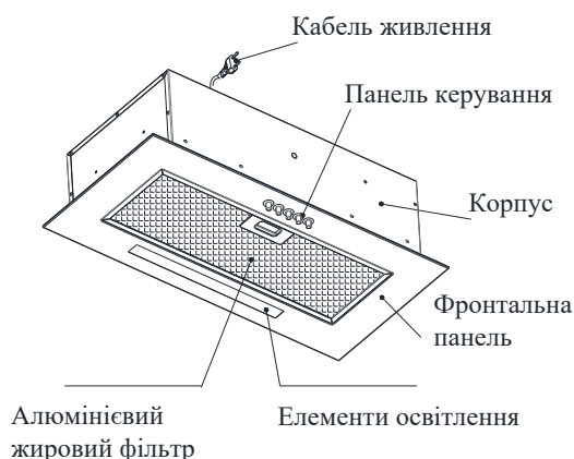
Рис. 1. Оглядове креслення кухонної витяжки
