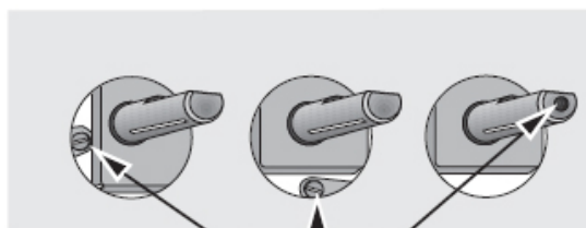
Обводной вентиль для регулировки минимального режима
