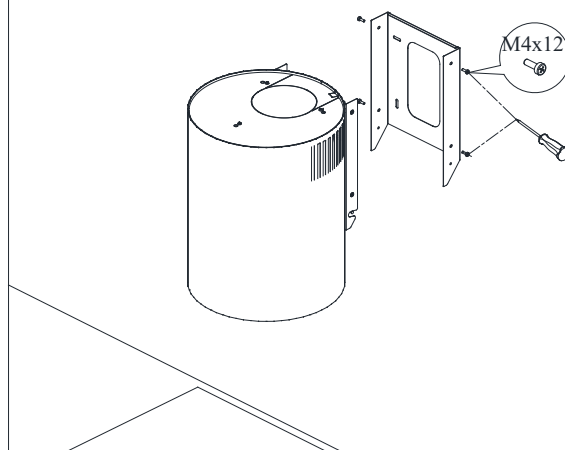
Рис. 8. Встановлення кухонної витяжки (присінний варіант монтажу)
