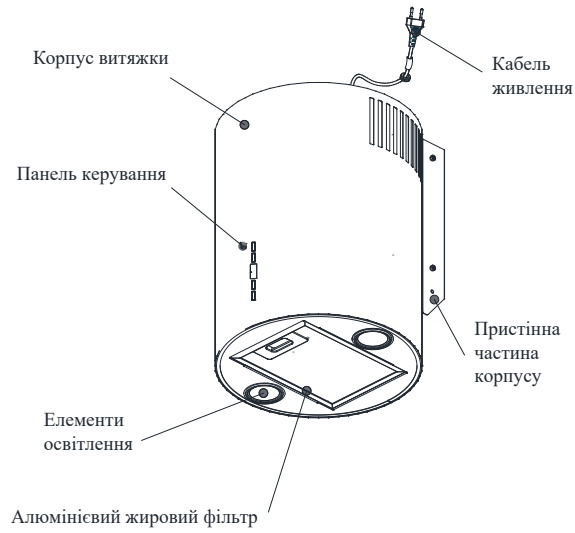
Рис. 1. Оглядове креслення кухонної витяжки
