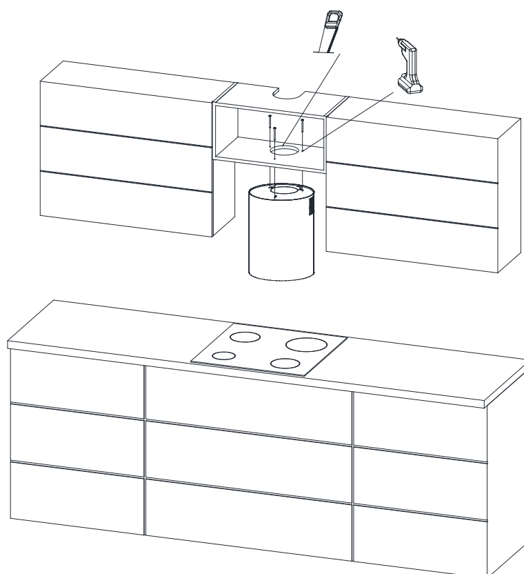
Рис.10. Монтаж витяжки під шафу
