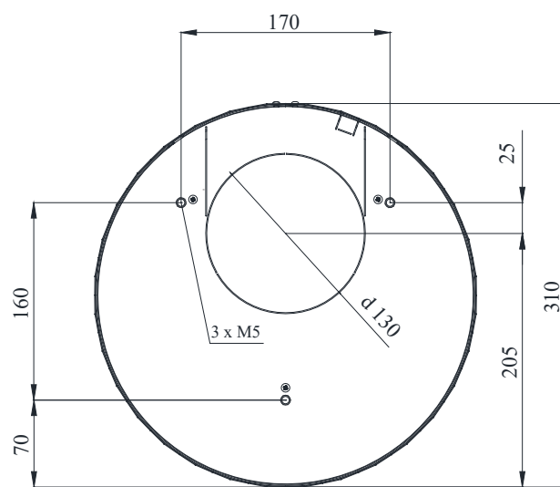
Рис. 3. Розміри монтажних отворів зверху
