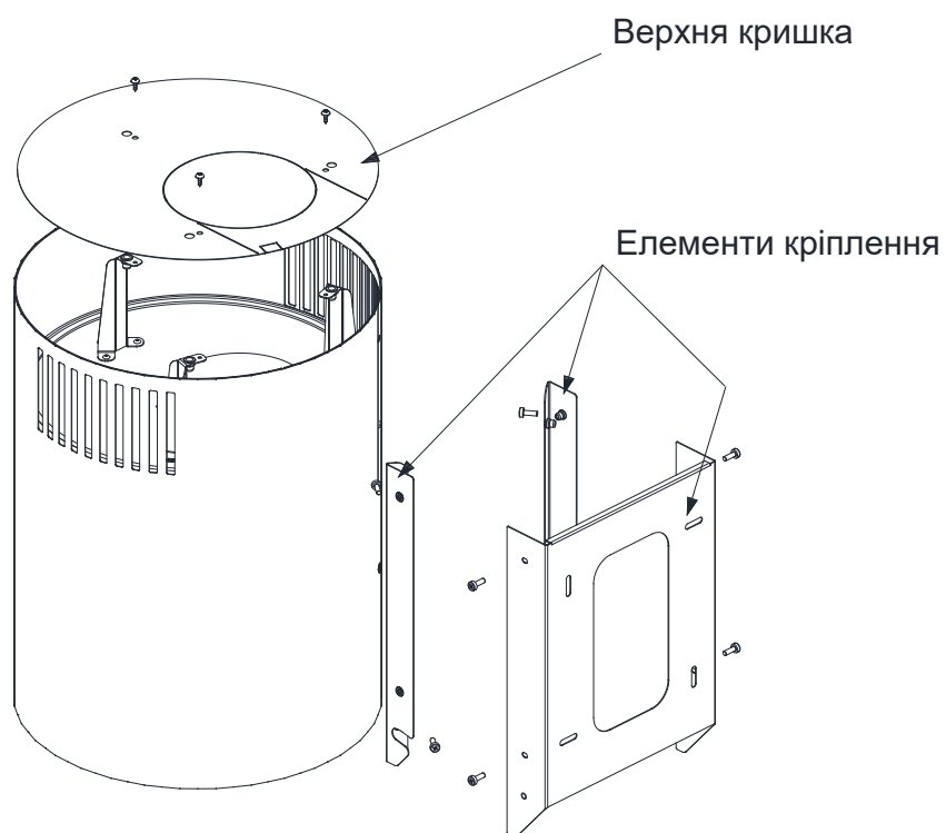
Рис.9: Демонтаж настінного кріплення
