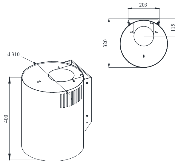
Рис. 2. Схема з розмірами моделі
