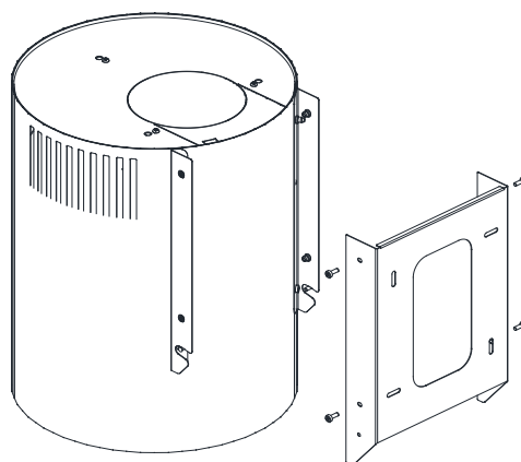
Рис. 6. Демонтаж кріплення
