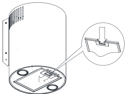
Рис. 11. Зняття алюмінієвого жирового фільтра
