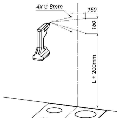
Рис. 5. Свердління монтажних отворів
