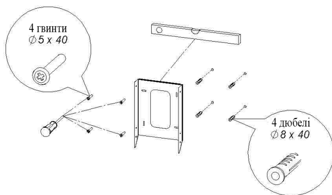
Рис. 7. Монтаж кріплення
